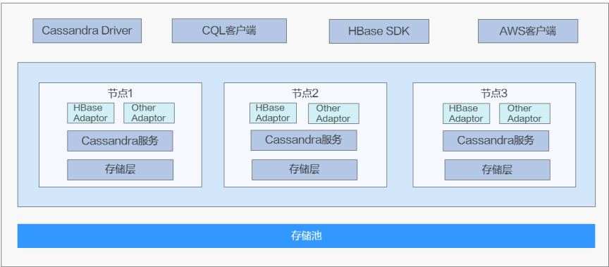
图 1-1 GeminiDB HBase 接口架构图
